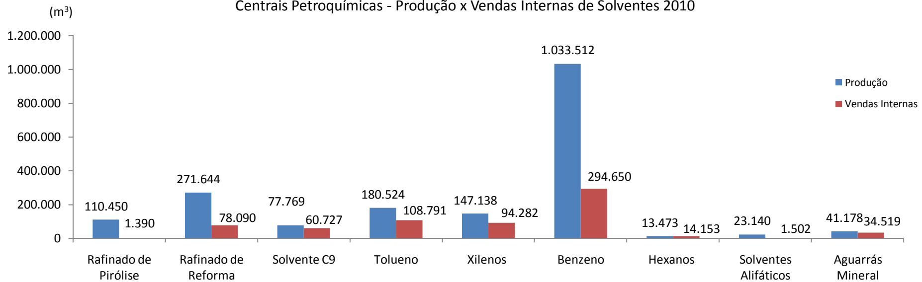
Centrais Petroquímicas - Produção x Vendas Internas de Solventes 2010
